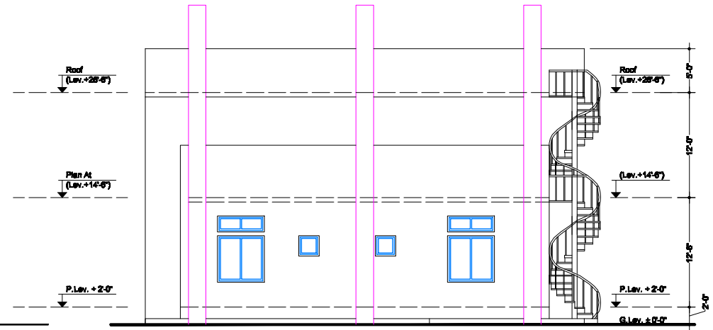
ELEVATION - 04
