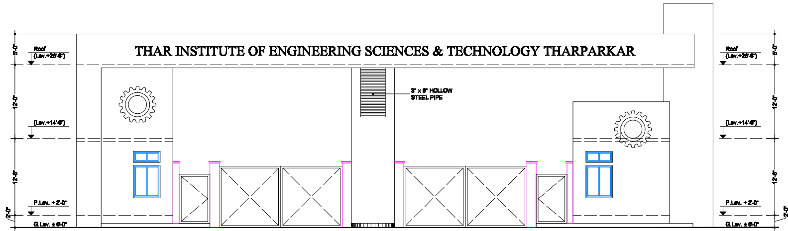
ELEVATION - 01
