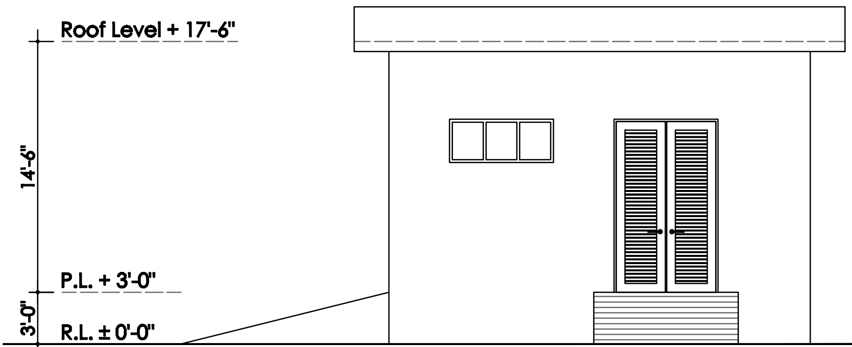
ELEVATION -02
