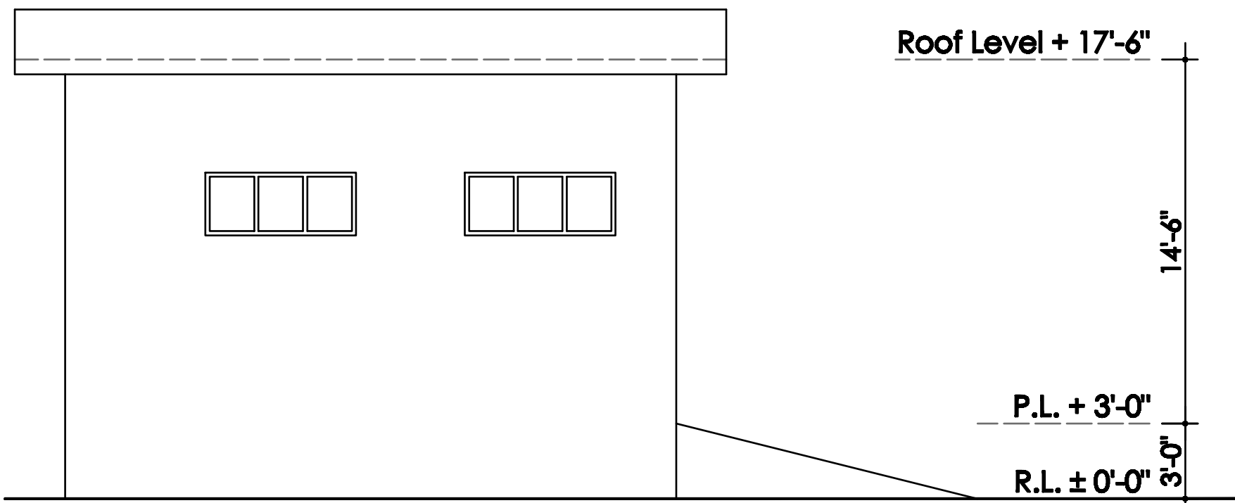
ELEVATION -04
