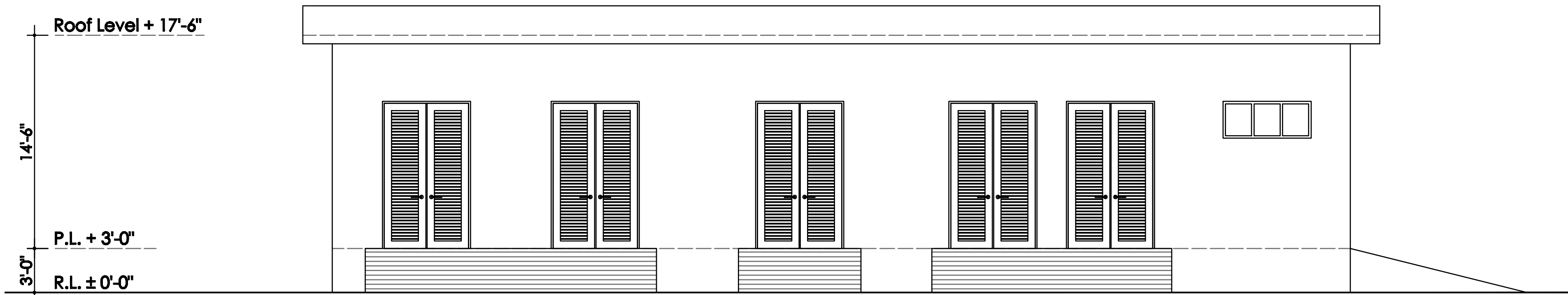
ELEVATION -01
