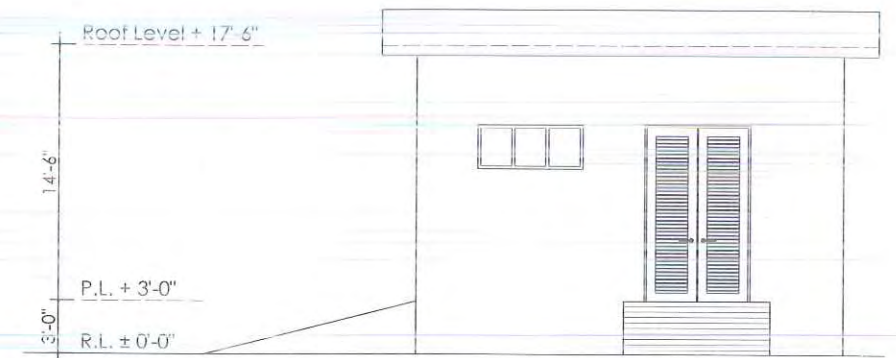
ELEVATION -02
