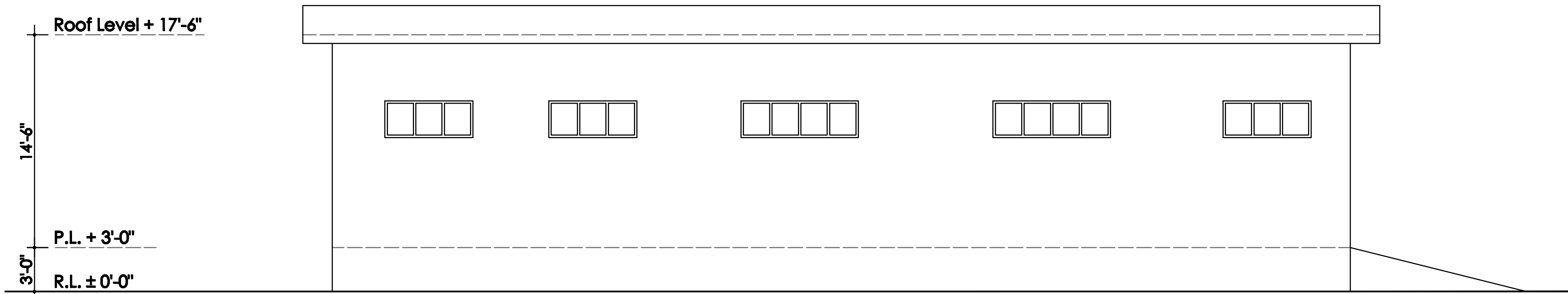
ELEVATION -03
