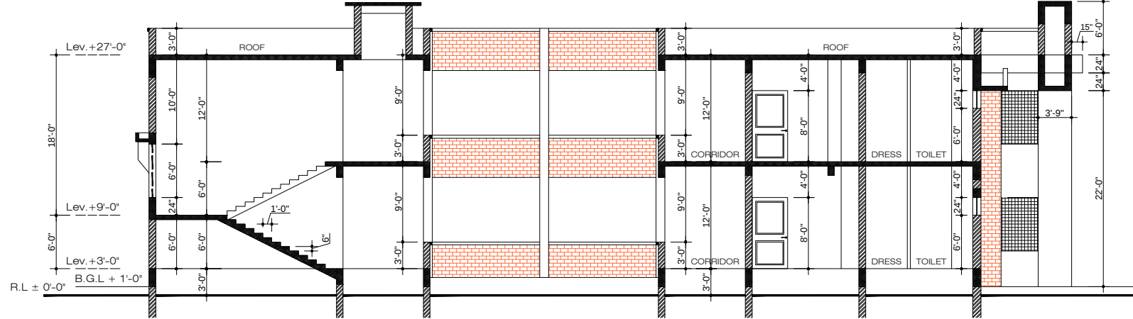
SECTION D-D
