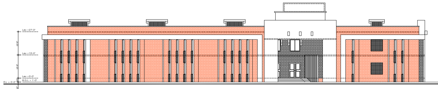
ELEVATION -04
