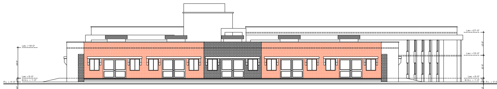
ELEVATION -02
